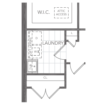
OPT. LAUNDRY IN LIEU OF LINEN A
