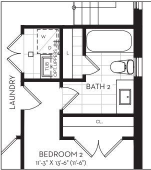
OPT. LAUNDRY IN LIEU OF W.I.L.
